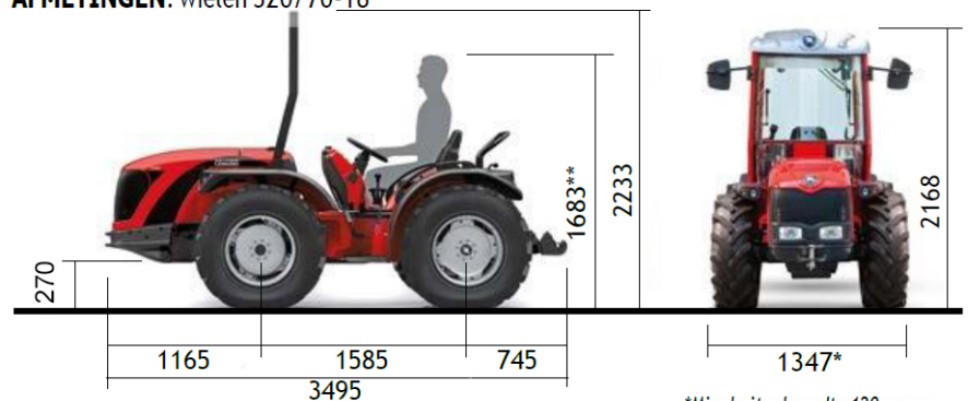
AFMETINGEN: wielen 320/70-18
